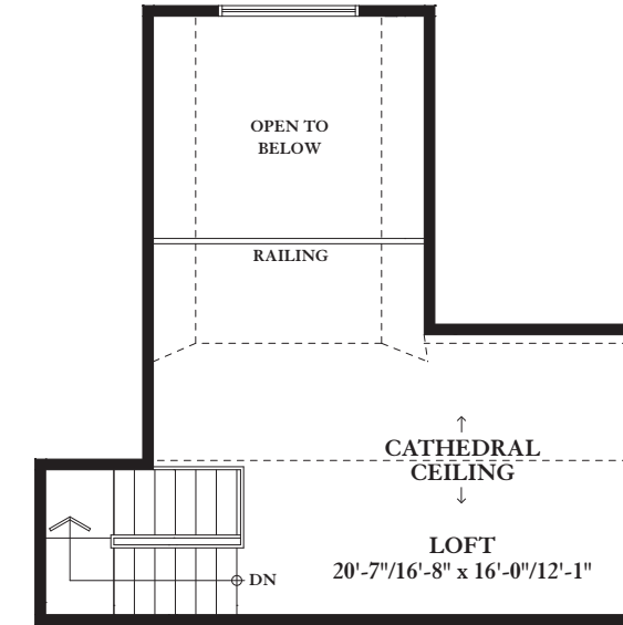
Optional Loft
